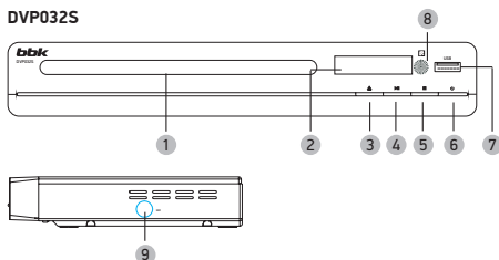
Рис. 1. Передняя и боковая панели DVD-плеера
