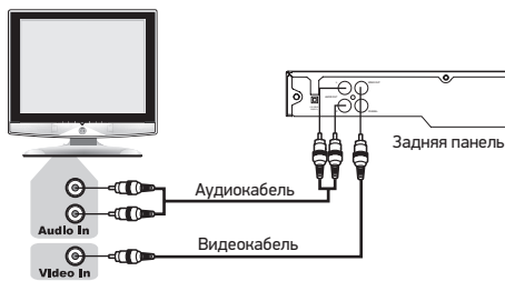
Рис. 3. Подключение к телевизору
